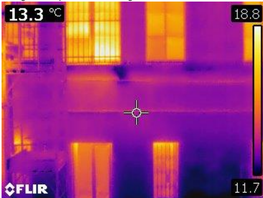
Figura 2.1 – Immagine termografica facciata - solaio interpiano
